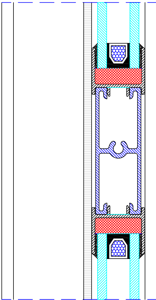
CORTE I
