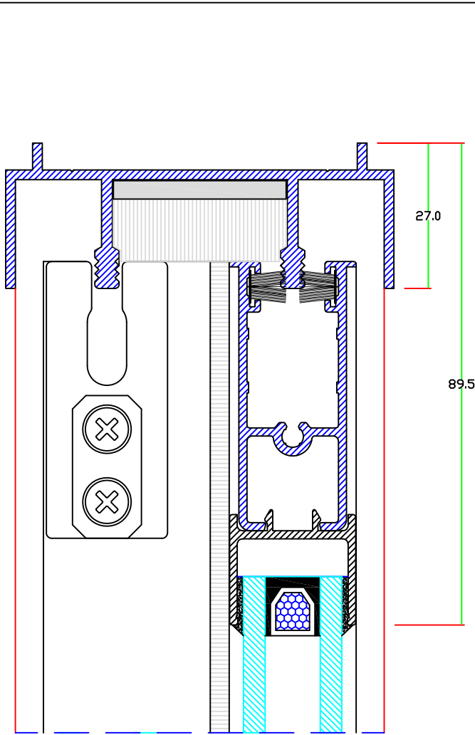
CORTE C
