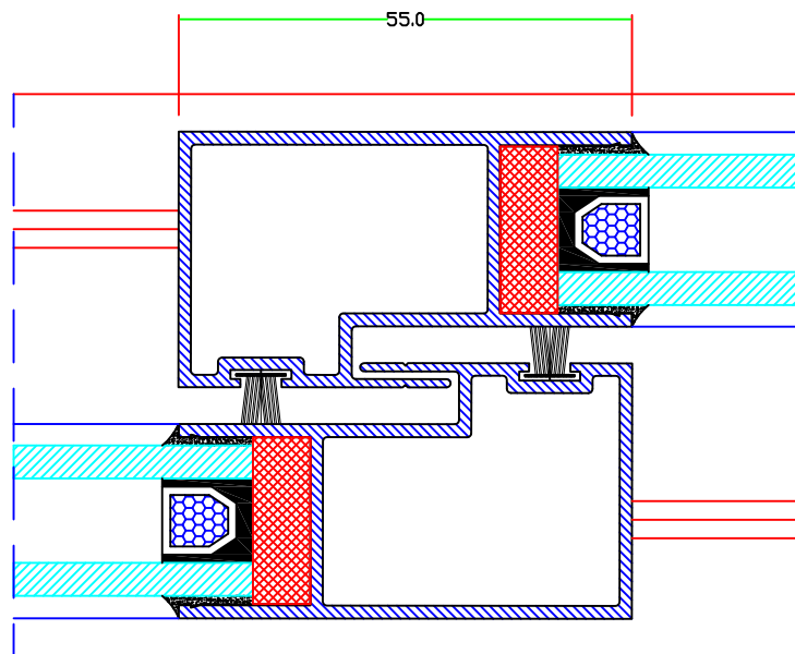
CORTE D
